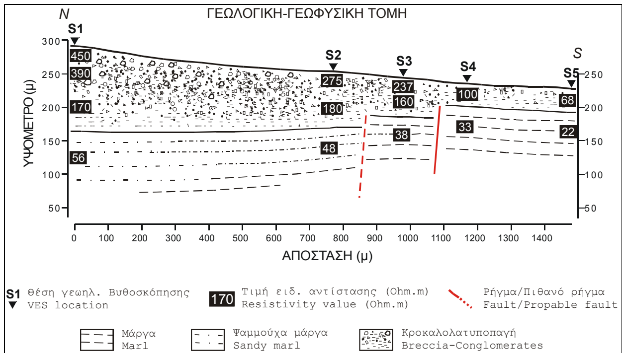
Εικόνα 5. Γεωλογική τομή, όπως προέκυψε μετά την εκτέλεση των γεωηλεκτρικών βυθοσκοπήσεων, σε κλίμακα 1:2. Figure 5. Geological section based on geophysical results, in scale 1:2.
