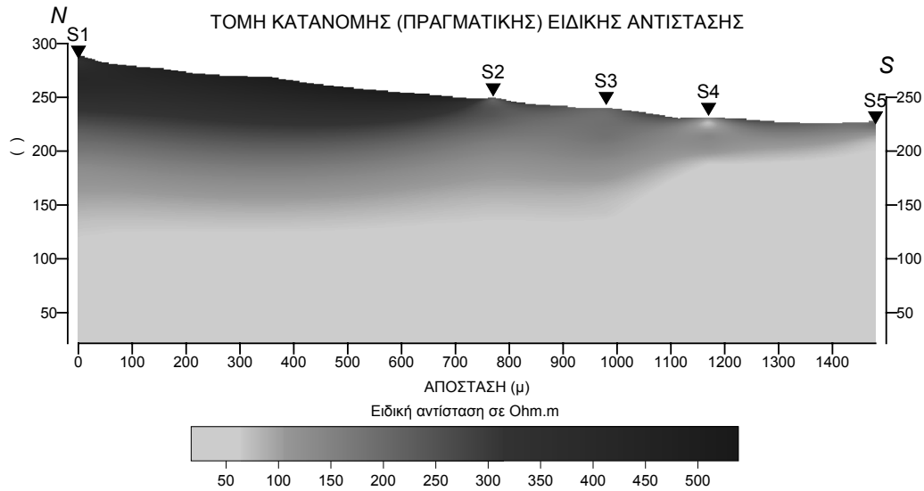
Εικόνα 4. Τομή κατανομής της (πραγματικής) ειδικής αντίστασης μετά του βάθους, σε κλίμακα 1:2. Figure 4. Resistivity cross-section, in scale 1:2.
